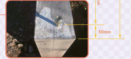
※アンカーボルト(ワッシャー1枚、ナット2個含む)は先行出荷が可能です。ご希望の際はお問い合わせください。 アンカーボルトはM10×160です。M12(市販品)も使用出来ますが、クリアランスに余裕が無い為、より本体施工精度が求められます(M12アンカーボルトをご使用の際は、ワッシャー(1枚)とナット(2個)もご用意ください。)
